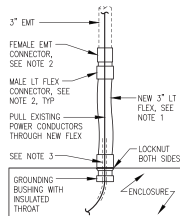
3 GENERATOR POWER CONDUIT CONNECTION E3.5 NO SCALE
